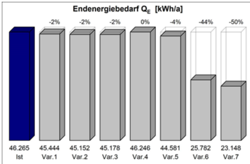
Abbildung 1 Endenergiebedarf Q_E [kWh/a]
