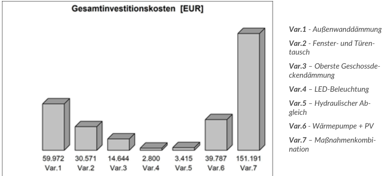
Abbildung 5 Gesamtinvestitionen [€]
