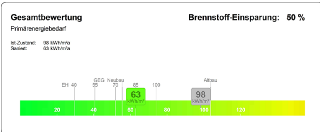
Abbildung 24 Gesamtbewertung Primärenergiebedarf, MK 1
