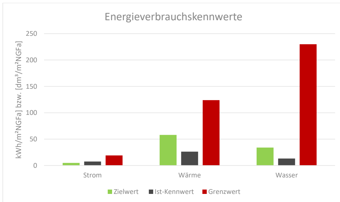
Abbildung 9 Grafische Darstellung der Energieverbrauchskennwerte
