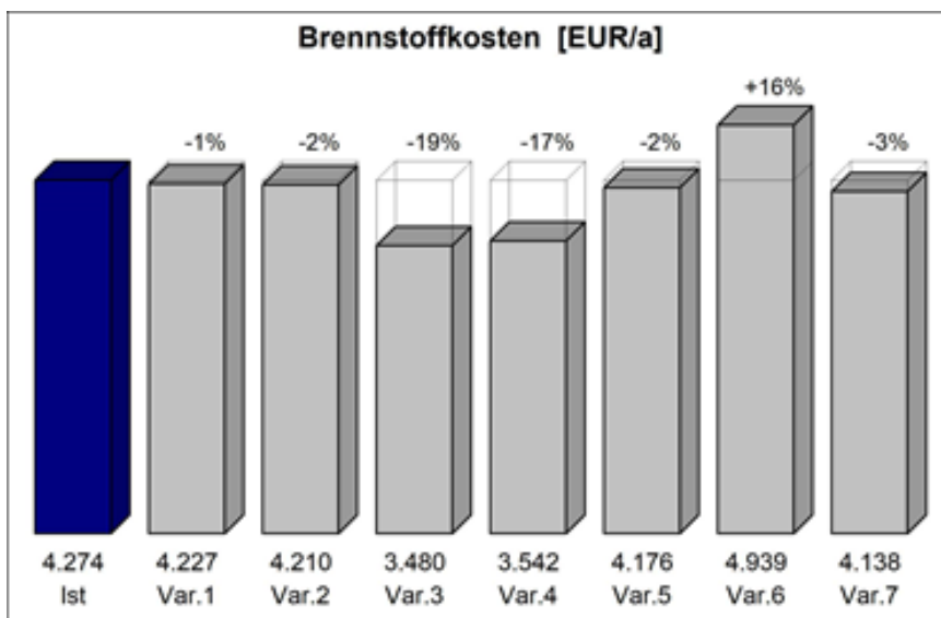
Abbildung 2 Brennstoffkosten [€/a]
