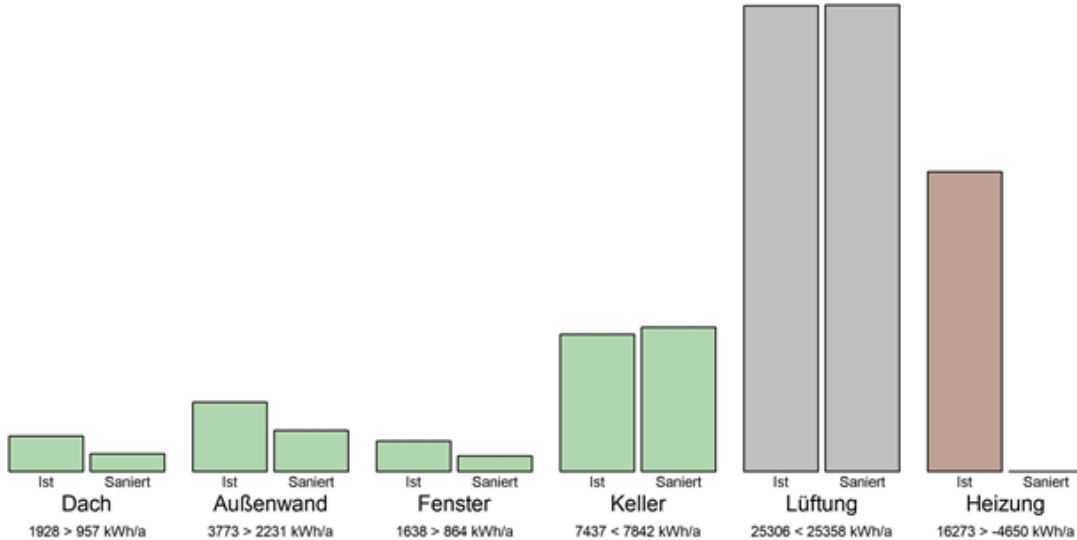
Abbildung 23 Einfluss der Sanierungsmaßnahme auf die Wärmeverluste [kWh/a], MK 1
