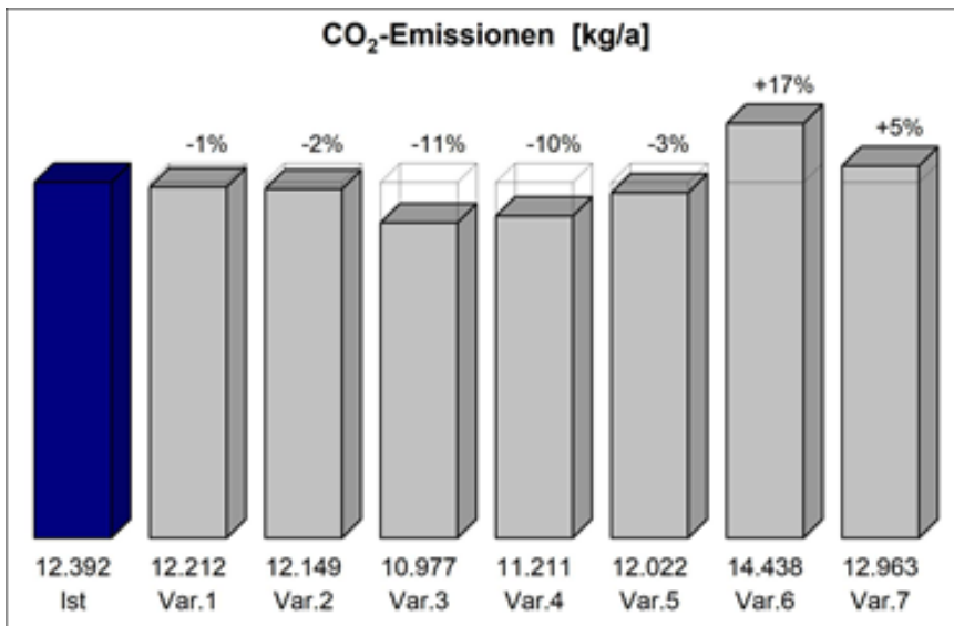
Abbildung 4 CO 2 -Emissionen [kg/a]
