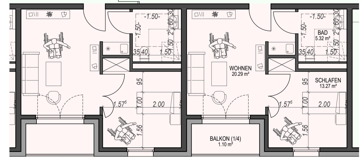
2.Obergeschoss Darstellung mit 37 Pflege-Appartments (ca. 40m²) (Ausstattung mit Kühlschrank, Spüle und Wasserkocher)
