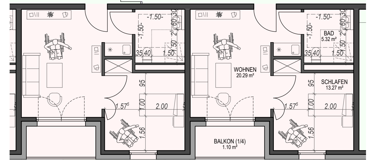
1.Obergeschoss Darstellung mit 37 Pflege-Appartments (ca. 40m²) (Ausstattung mit Kühlschrank, Spüle und Wasserkocher)
